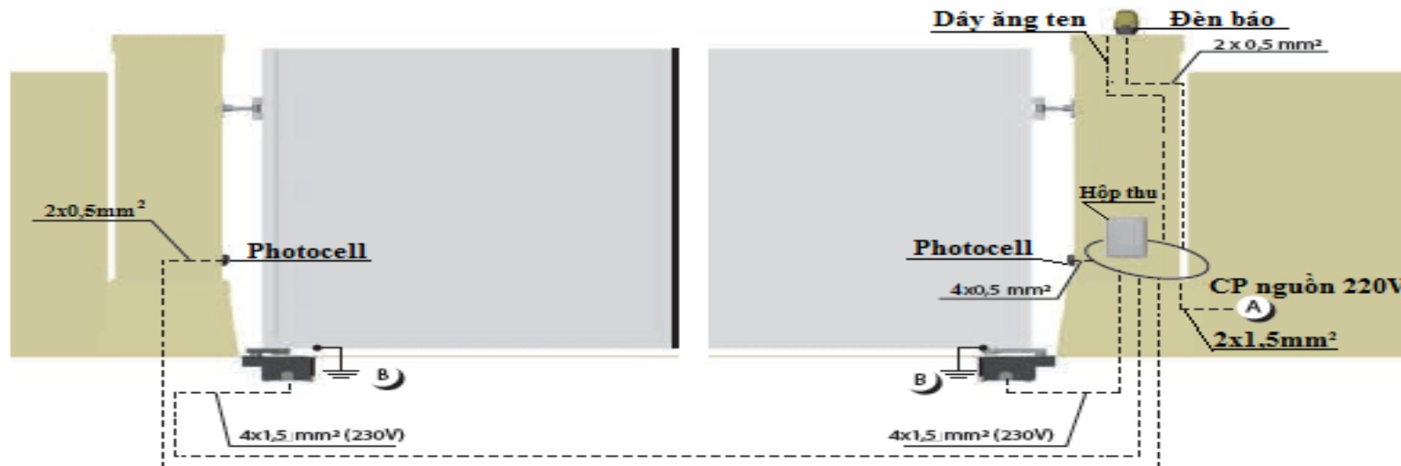
Sơ Đồ Đi dây điện Motor GHOST 200-220V
