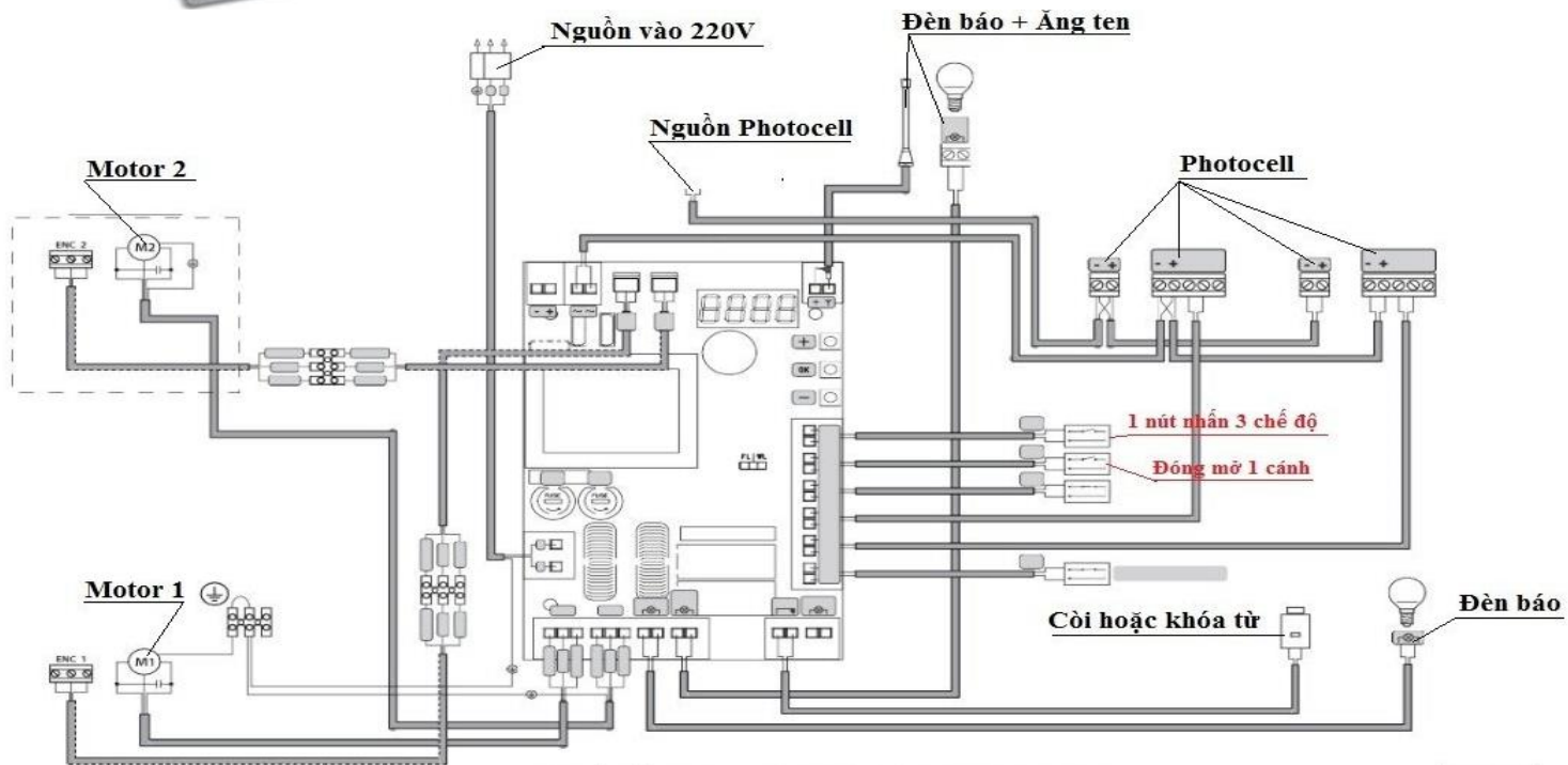
Sơ Đồ Đấu Dây Cho Motor GHOST 200- 220V
