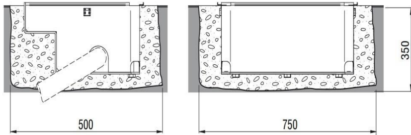
Kích thước hố Bê tông chôn hộp để
