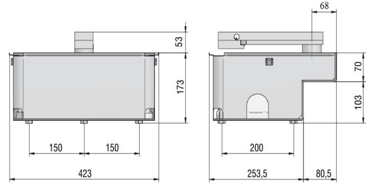
Kích thước hộp để
