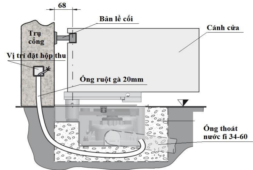
Quy Cách Đặt Hộp Chôn Nền
